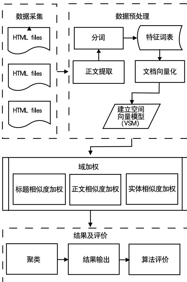
图1 系统流程图
